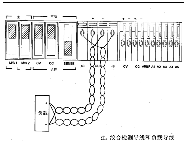
图 5，远程电压检测
