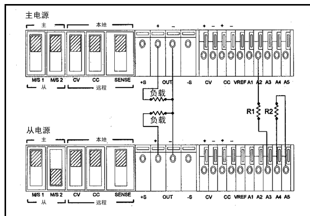
图 14, 两个电源的自动跟踪操作
